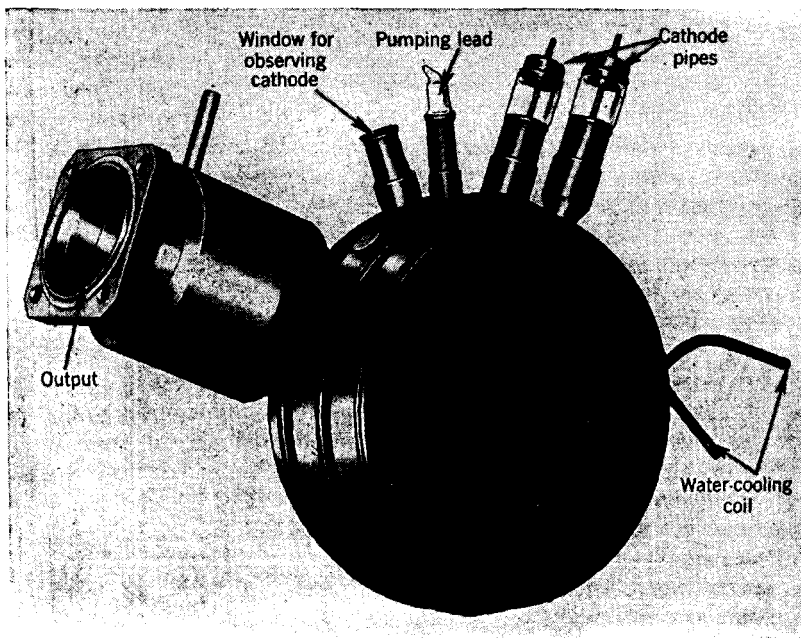
Fig. 19-6.—LCW magnetron.
